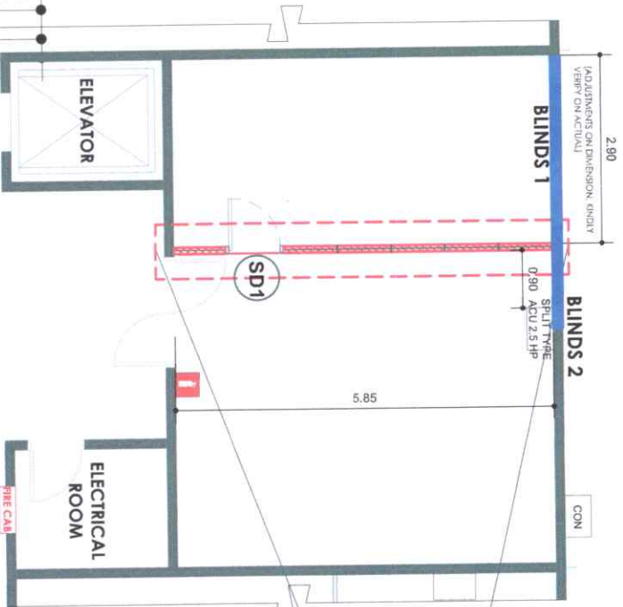
FLOOR PLAN SCALE: 1:100M
